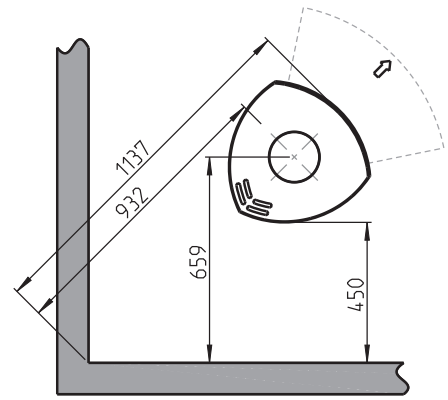
Min. distance to combustible wall
