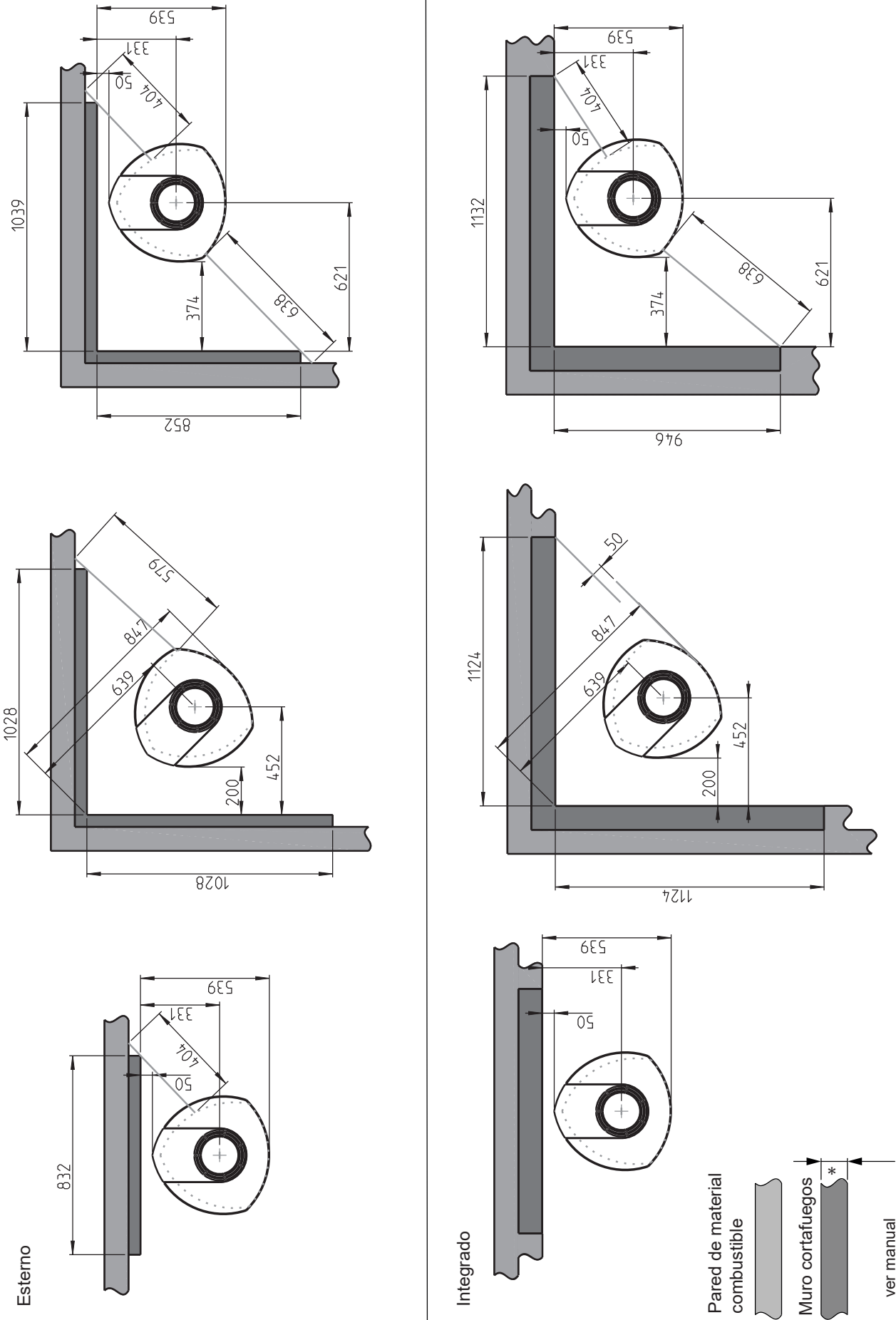
Jøtul F 377 Advance - Distancia mínima a una pared de material no combustible
