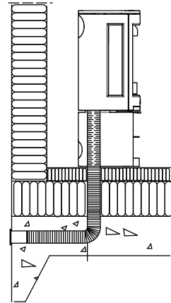
Fig. 2C, attraverso il pavimento e il basamento
